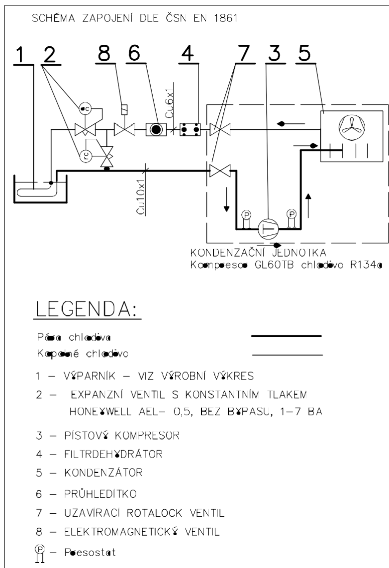
Obr. 1: Schéma zapojení chladicího okruhu
